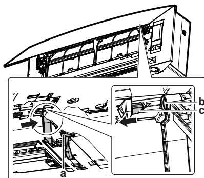
a Bras b Fente d'arbre c Arbre
