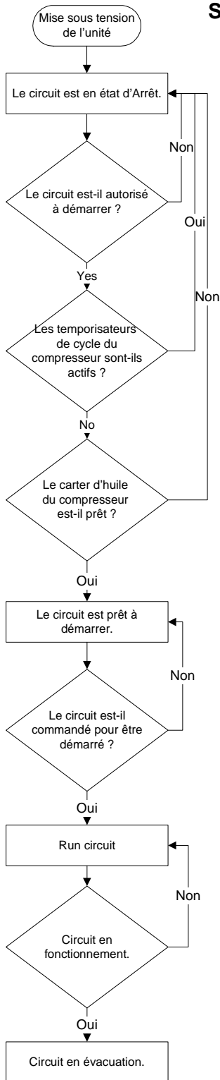
Figure 6 : séquence de fonctionnement du circuit
