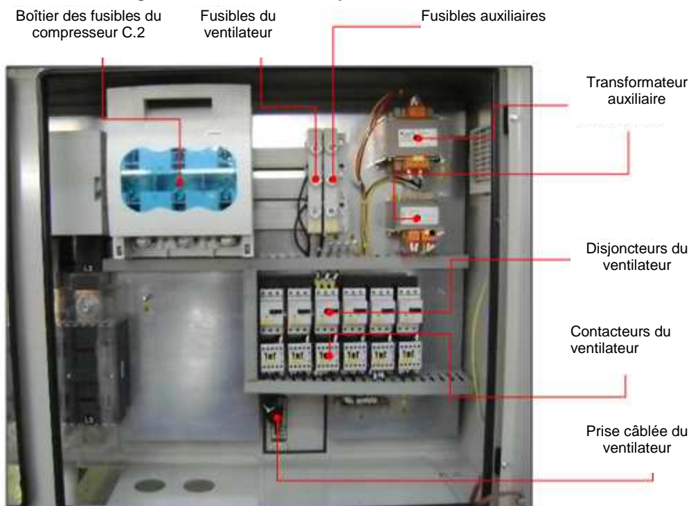
Figure 3 : tableau électrique, côté droit
