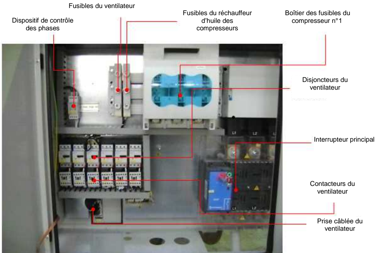
Figure 2 : tableau électrique, côté gauche
