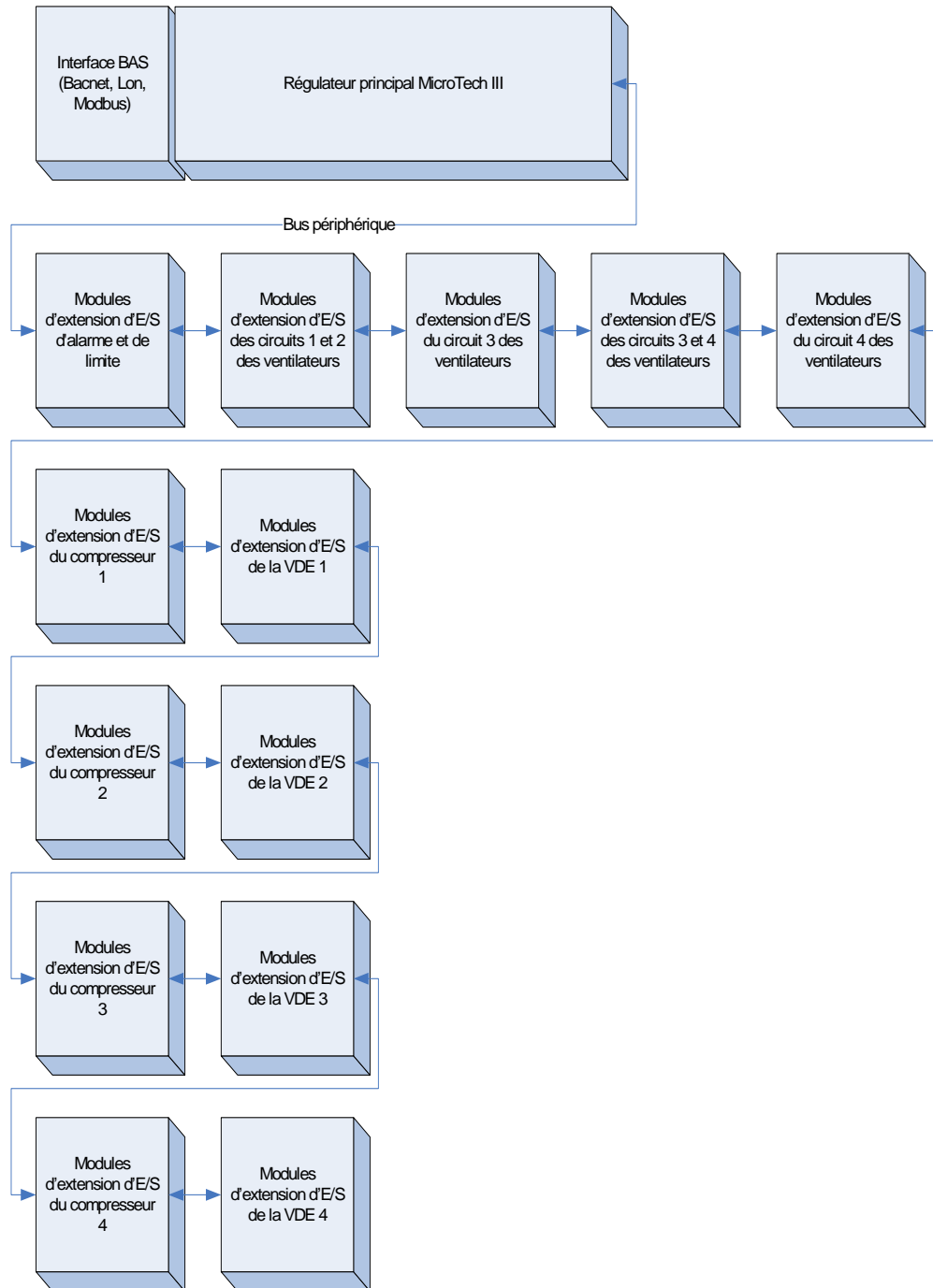
Figure 4 : architecture du système
