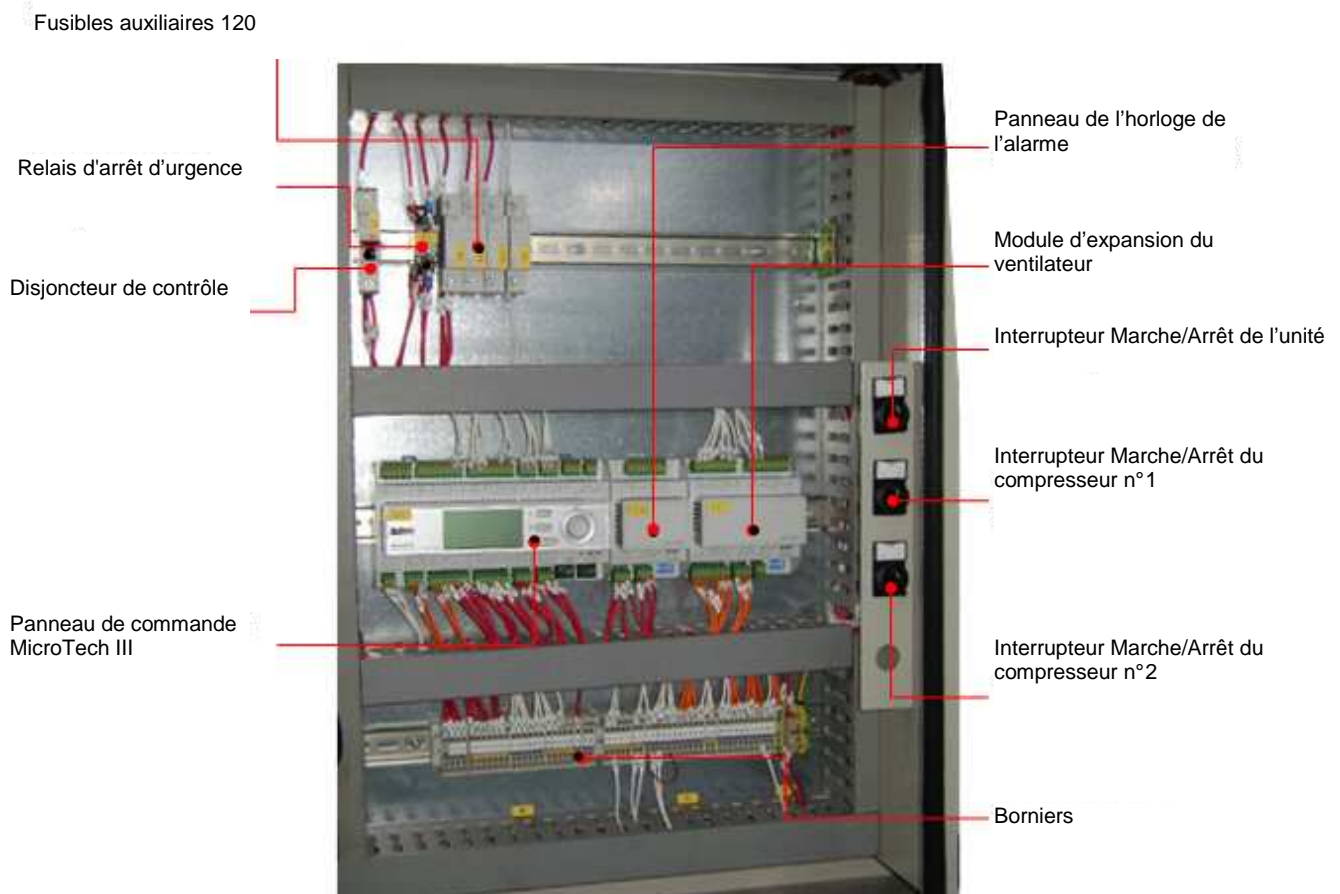
Figure 1 : composants du panneau de commande
