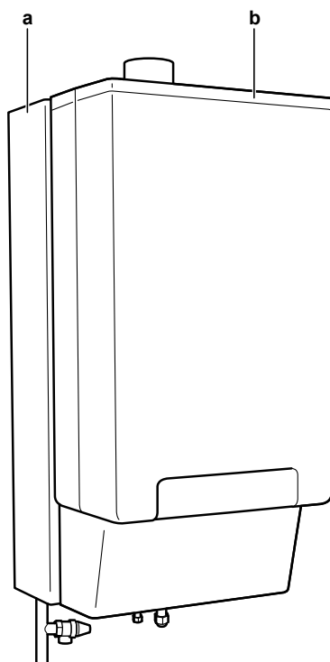
a Module pompe à chaleur b Module de chaudière à gaz
