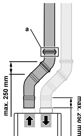
a 2 e élément après le 1 er coude
