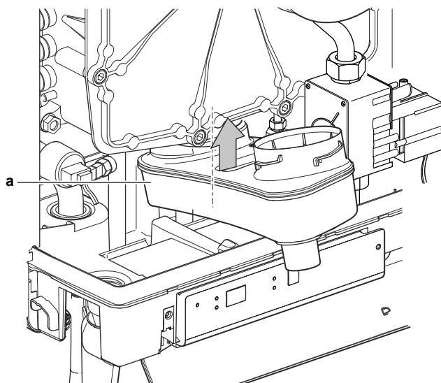
a Plateau de base
