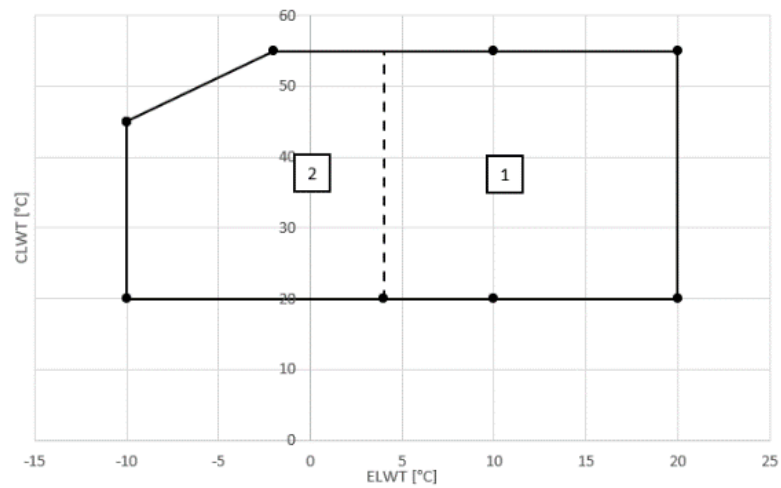
Figure 4- Plage de fonctionnement EWWQ049-064
