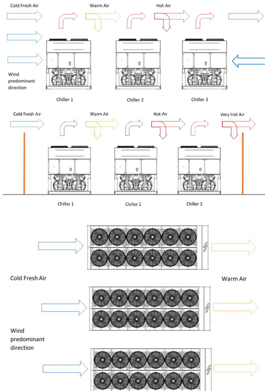
Figure 7- Installation de refroidisseurs multiples
