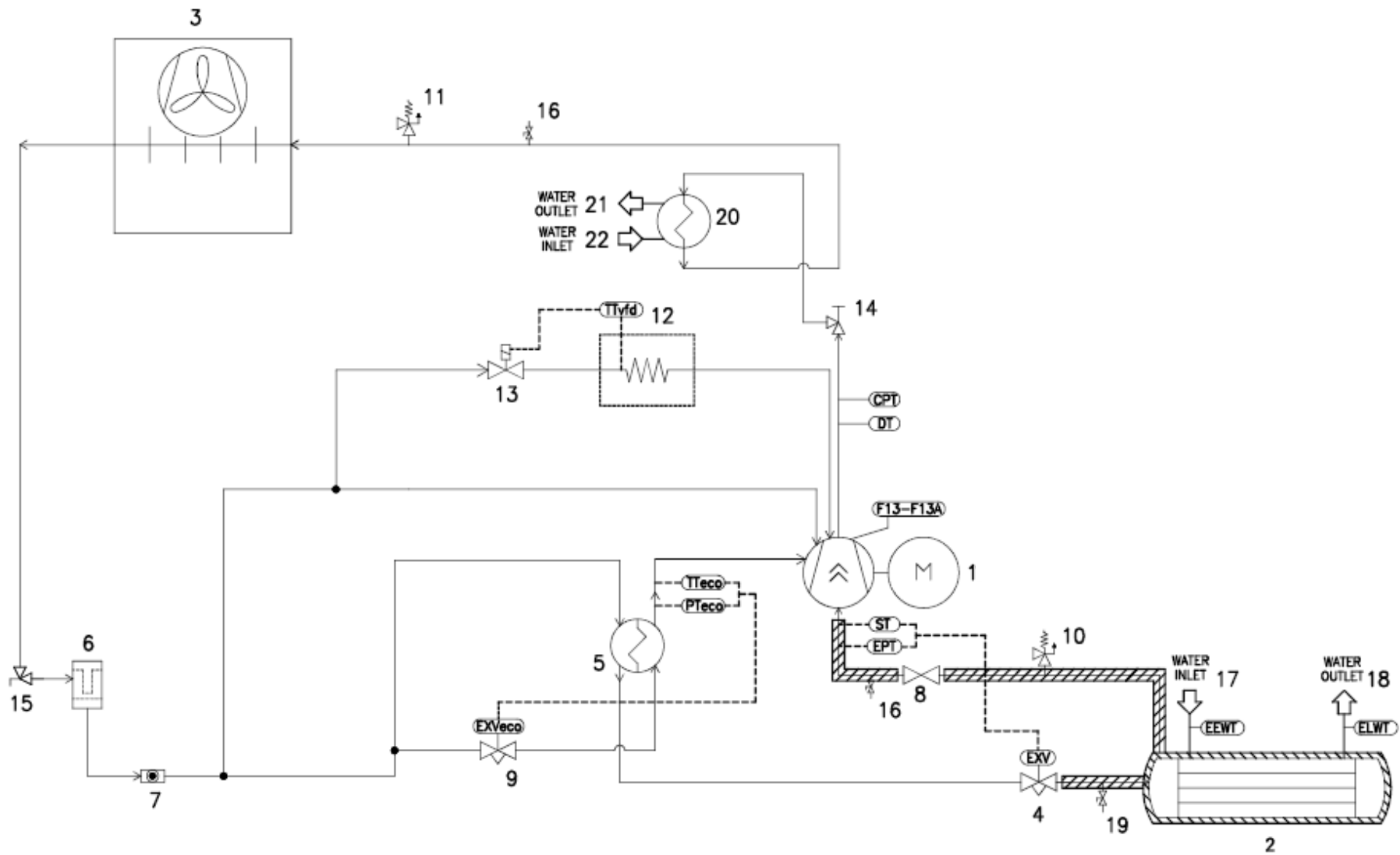
Figure 2 - Circuit réfrigérant standard avec récupération de chaleur
