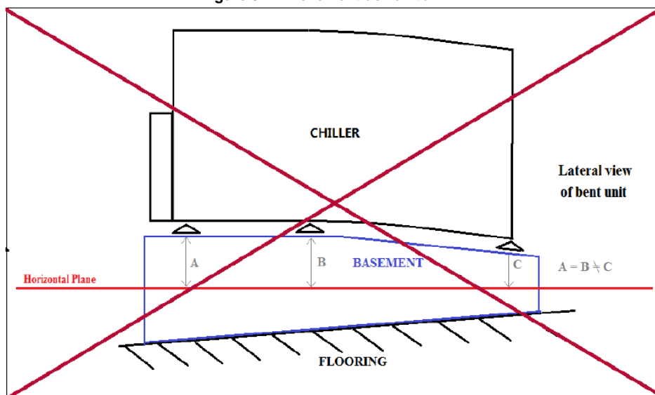
Figure 5 – Nivellement de l'unité
