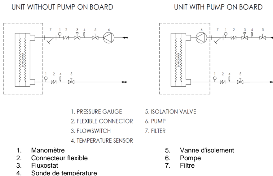
Figure 9 - Raccordement des tuyaux d'eau pour les échangeurs de récupération de chaleur
