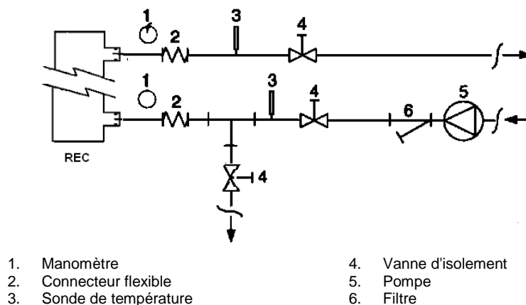
Figure 9 - Raccordement des tuyaux d'eau pour les échangeurs de récupération de chaleur
