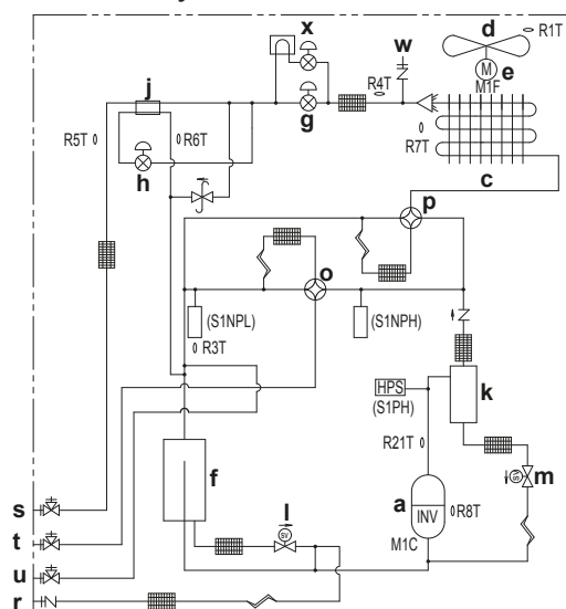
Schéma des tuyauteries : RYMQ8~12
