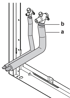
a Matériau d'isolation b Matage, etc.
