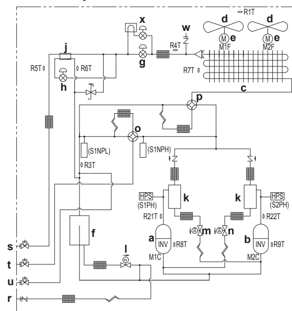
Schéma des tuyauteries : RYMQ14~20
