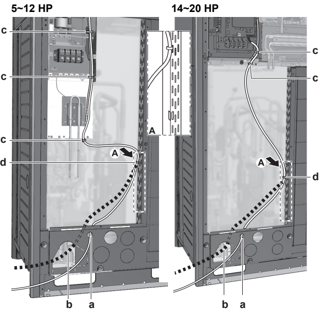
a Ligne d'interconnexion (possibilité 1)(a)
