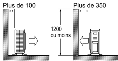
Mur faisant face à un côté
