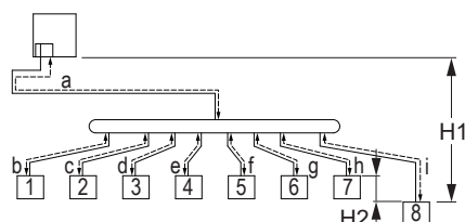
18-3 Exemple 3: en cas de collecteur refnet uniquement
