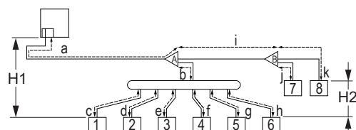
18-2 Exemple 2: en cas de raccords refnet et de collecteur
