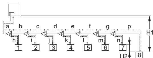
18-1 Exemple 1: en cas de raccords refnet uniquement
